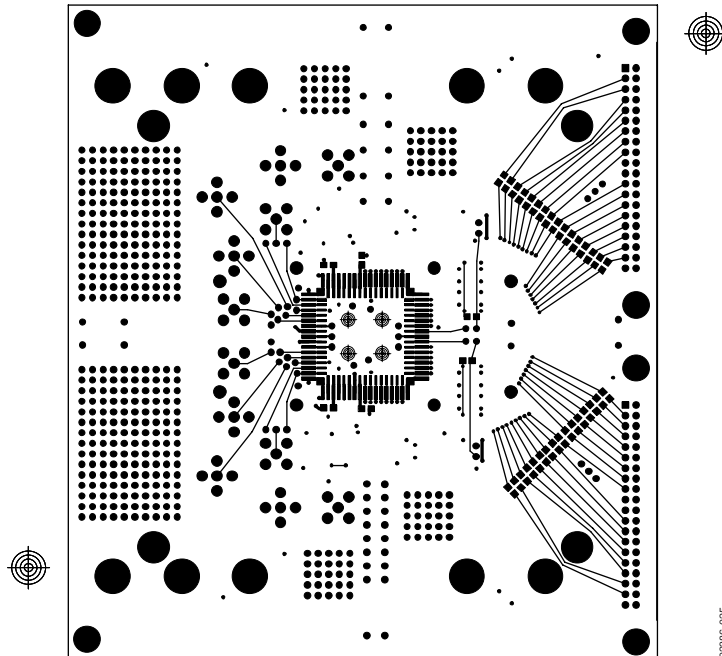
Figure 25. Top Layer
